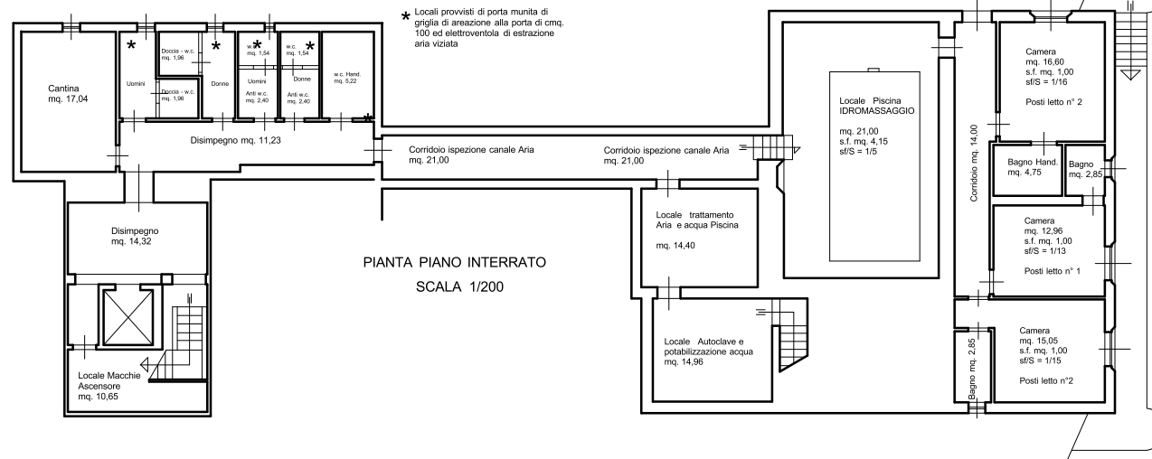
PIANTA PIANO INTERRATO EDIFICIO PRINCIPALE
