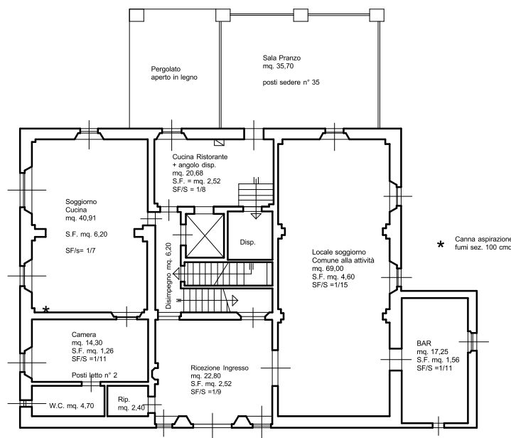
PIANTA PIANO TERRA EDIFICIO PRINCIPALE
